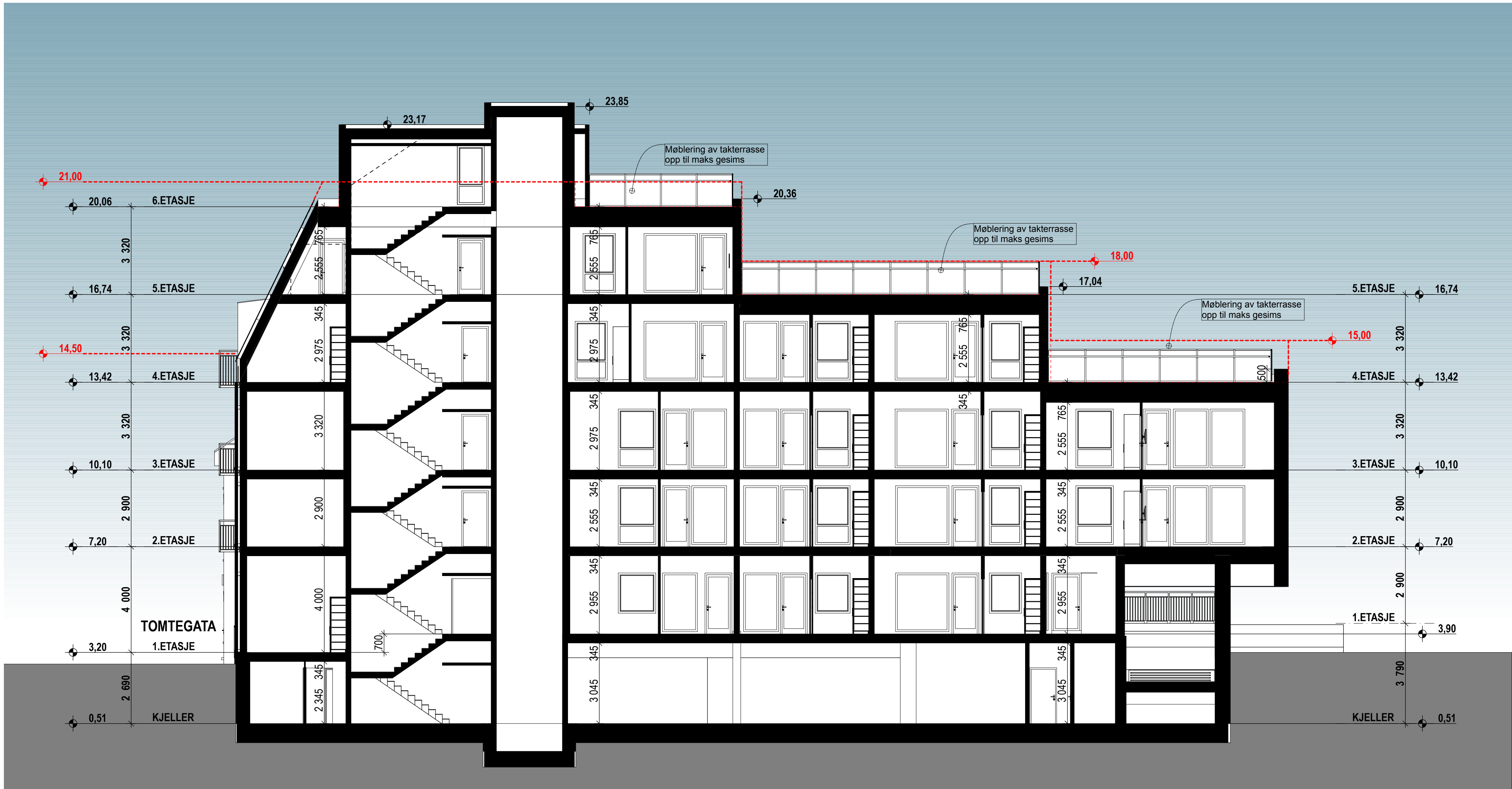
Snitt D
