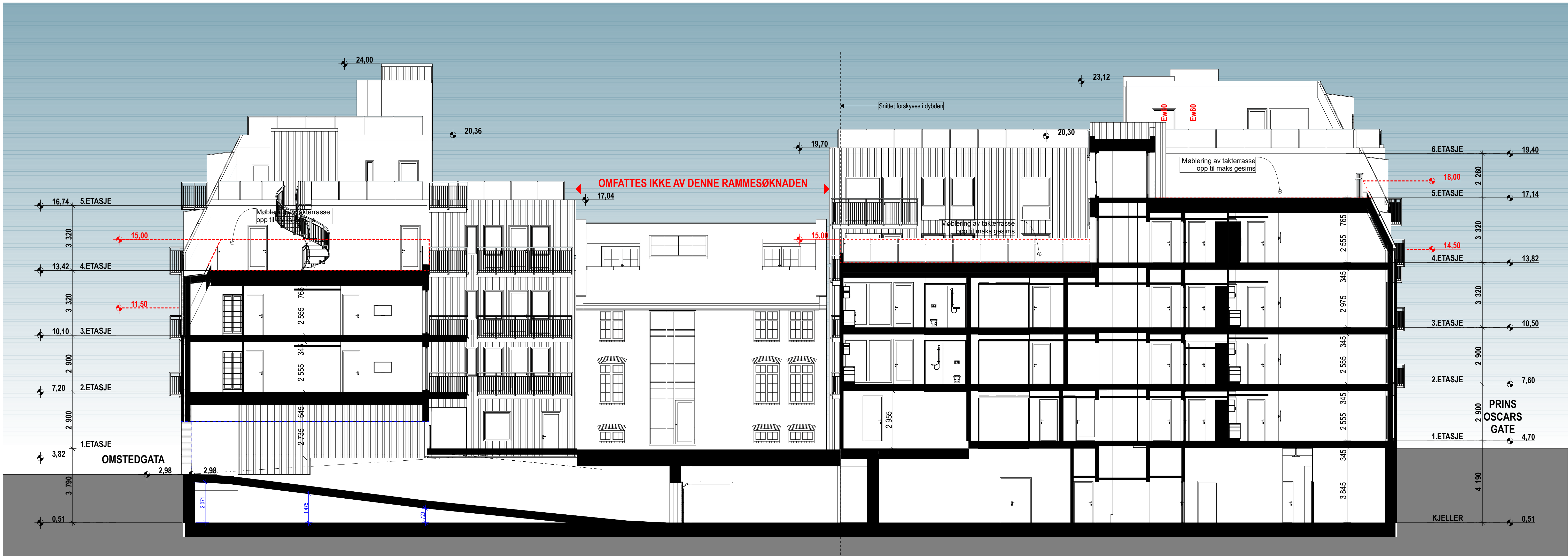
Snitt A
